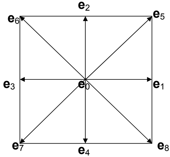
(a) D2Q9
